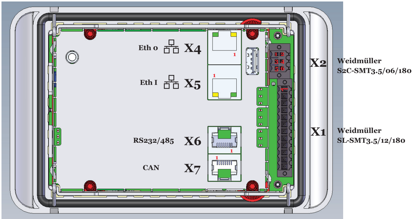
Abbildung 3: Anschlussbelegung
